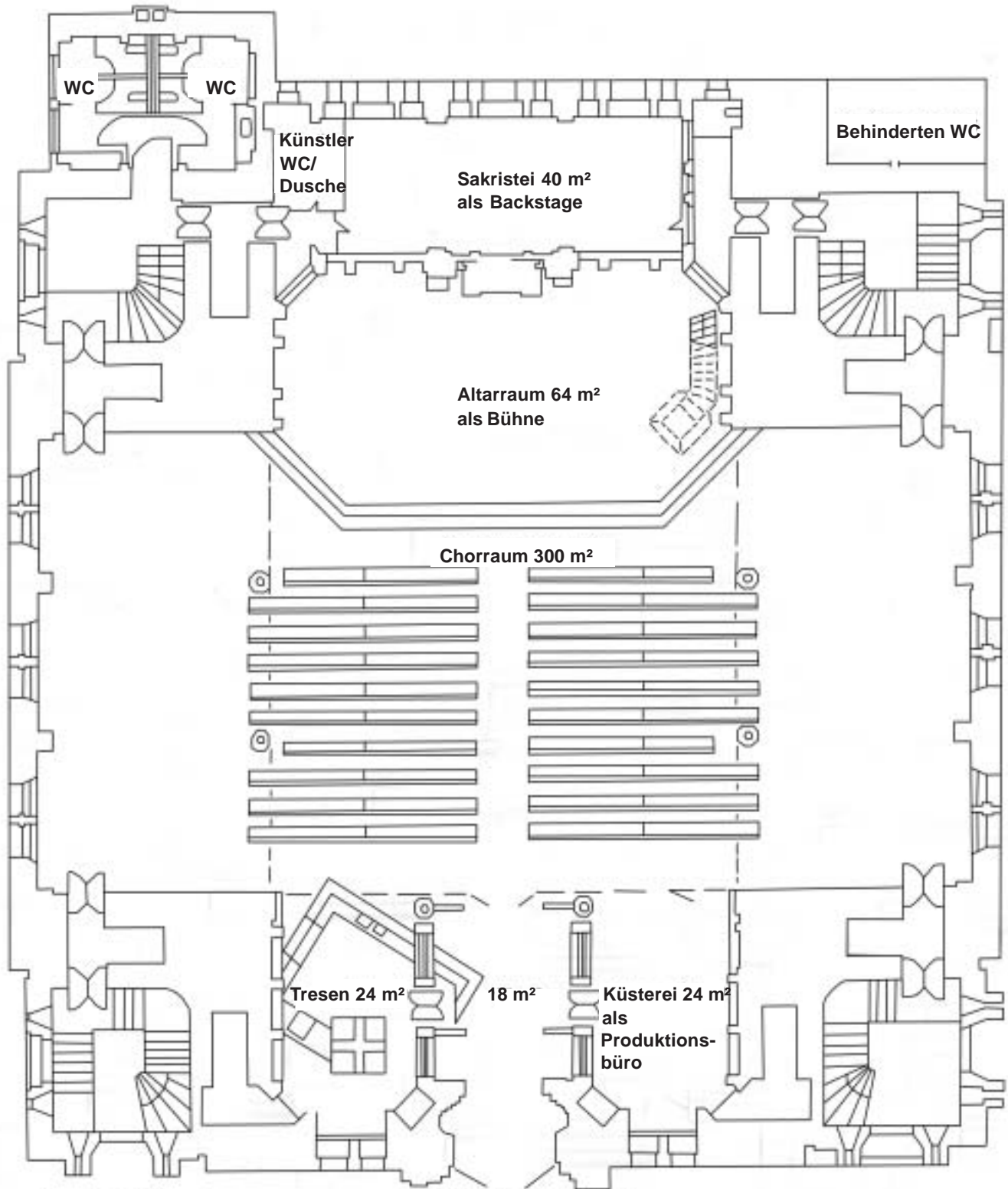
Grundriss Erdgeschoss
